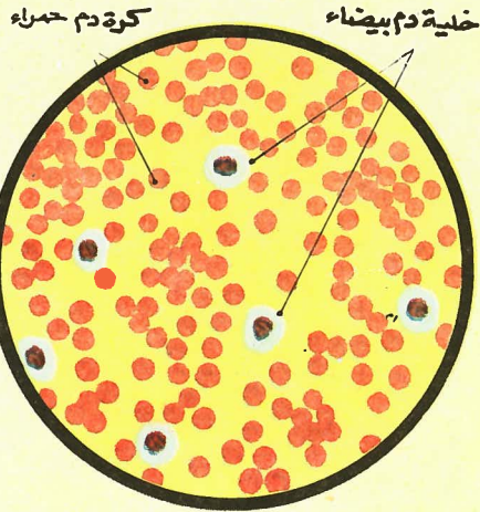
منظر لدم العادي تحت الميكروسكوب ( X - ٤٠٠ )
