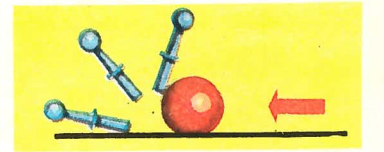
طاقة حركية أو طاقة الحركة
