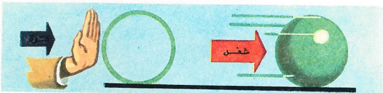
ينتج شغل نتيجة ندفة اليد
